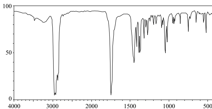
Spectre IR du produit obtenu
