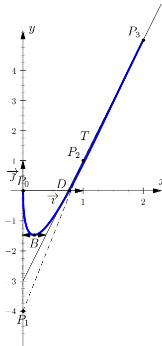
FIGURE 64.4 – Courbe de Bézier pilotée par les points A_0, A_1, A_2, A_3 donnés par l'énoncé
