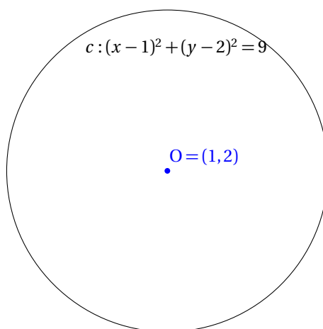
FIGURE 27.6 – Equation cartésienne d'un cercle de centre O(1, 2) et de rayon 3
