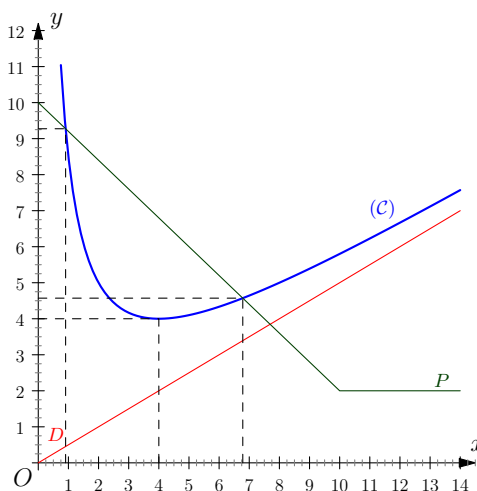
FIGURE 59.3 – Représentation graphique
