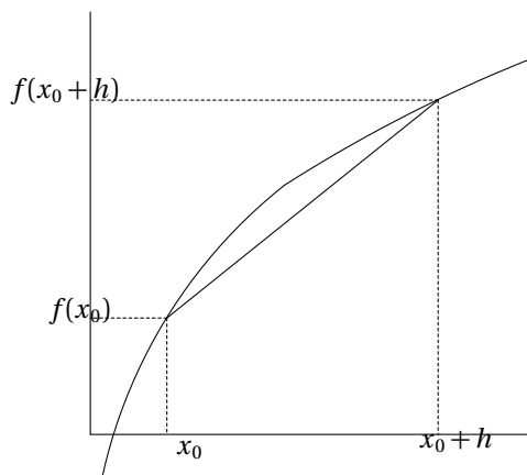
FIGURE 49.1 – Accroissement moyen de f
