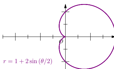
FIGURE 54.2 – Cardioïde
