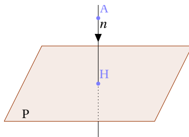
FIGURE 40.8 – Distance d'un point à un plan
