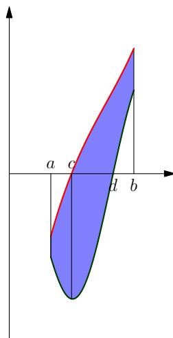
FIGURE 66.18 – Découpage des fonctions f et g selon leurs signes respectifs
