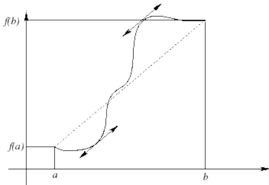
FIGURE 48.1 – Interprétation géométrique du théorème des accroissements finis
