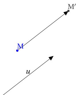
FIGURE 35.1 – Translation de vecteur u
