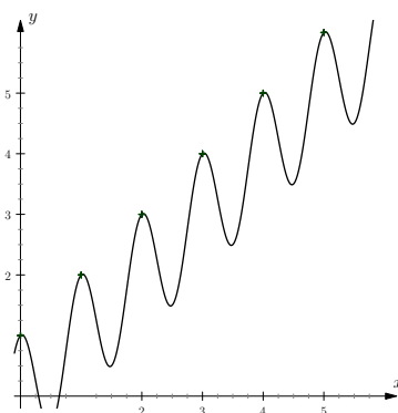
FIGURE 41.2 – La fonction f(x) = \cos(2\pi x) + x n'est pas croissante et pourtant, la suite u_n = f(n) est croissante
