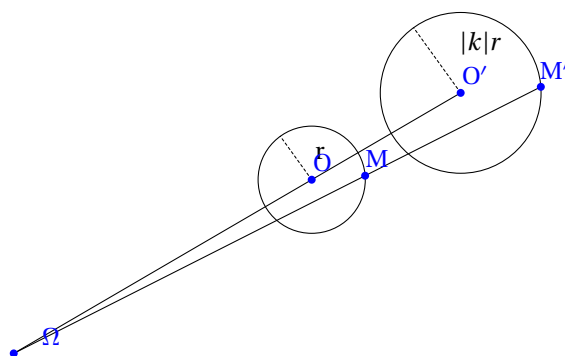
FIGURE 35.9 – L'image d'un cercle par une homothétie est un cercle
