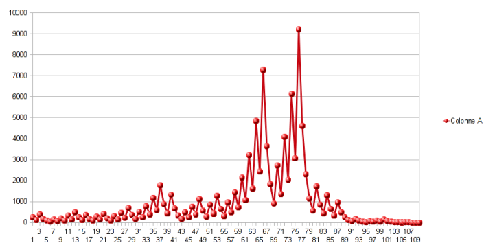
FIGURE 68.6 – Courbe représentative de la suite de Syracuse associée à a = 250
