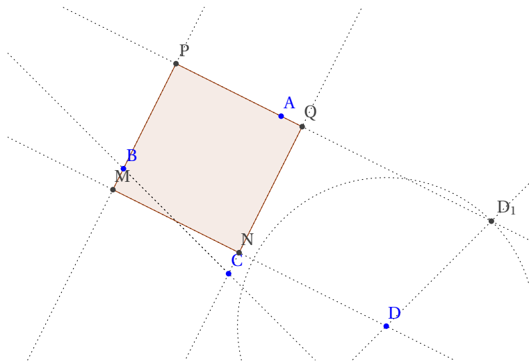
FIGURE 38.5 – Problème du carré passant par quatre points quelconques
