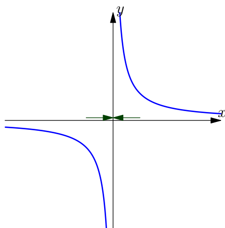
FIGURE 47.6 – Limite à gauche et à droite
