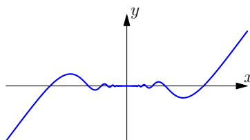
FIGURE 49.4 – Représentation graphique de la fonction f(x) = x^2 \sin \frac{1}{x} si x \neq 0 et f(0) = 0
