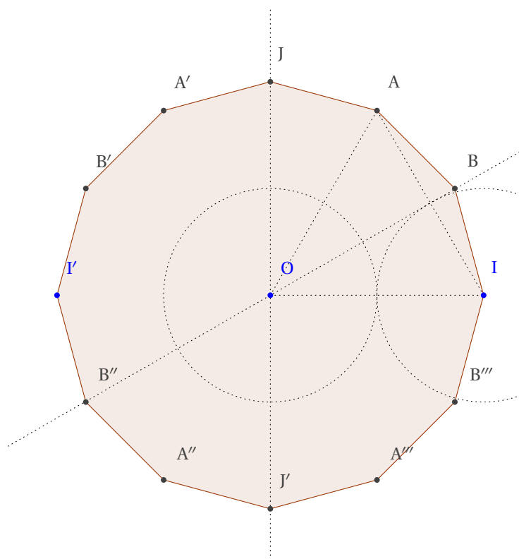
FIGURE 38.4 – Le dodécagone
