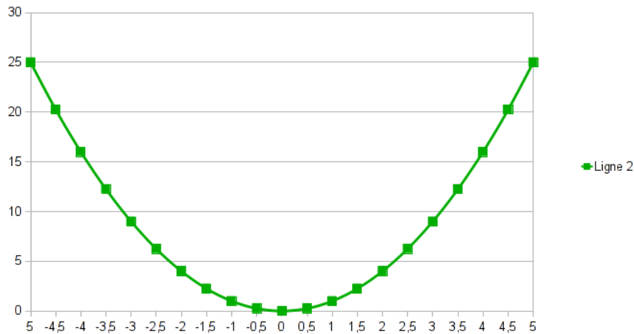
FIGURE 68.9 – Courbe représentative de la fonction f : x \mapsto x^2 sur l'intervalle [-5, 5]
