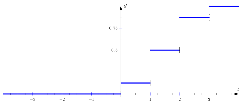
FIGURE 5.1 – Fonction de répartition de X
