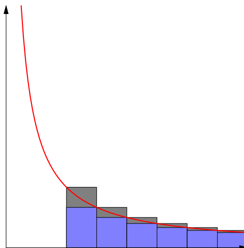
FIGURE 66.13 – Représentation des suites u_n et v_n
