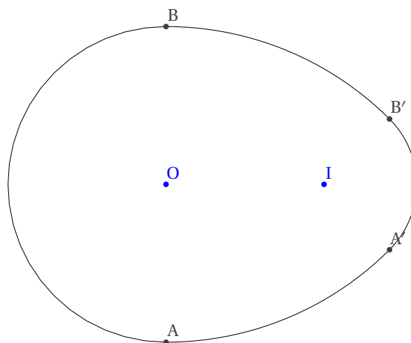
FIGURE 38.2 – Un oeuf
