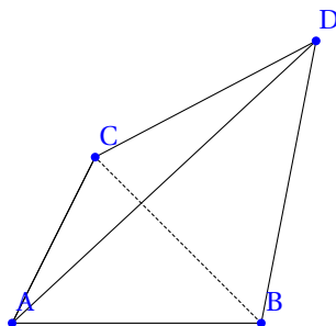
FIGURE 28.4 – Le tétraèdre
