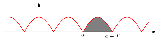
FIGURE 55.9 – Intégrales d'une fonction périodique
