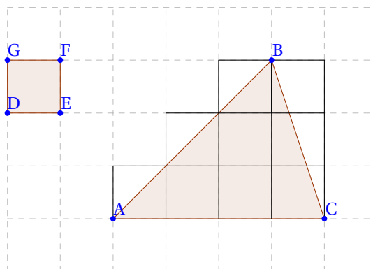
FIGURE 66.5 – Mesurer l'aire d'une figure
