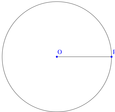
FIGURE 66.10 – L'aire du cercle de rayon 3 cm est 9\pi \text{ cm}^2
