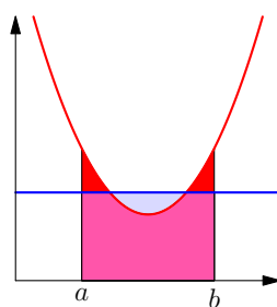
FIGURE 55.7 – Valeur moyenne
