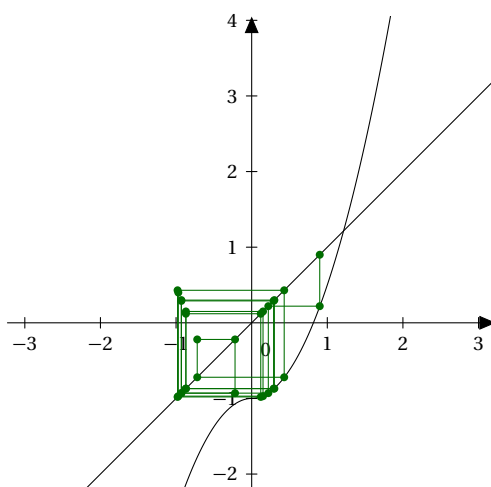
FIGURE 45.1 – Représentation graphique de la suite u_{n+1} = 1,5u_n^2 - 1 quand u_0 = 0,9
