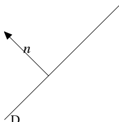
FIGURE 30.3 – Le vecteur n est normale à la droite D
