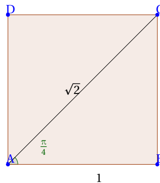
FIGURE 32.6 – Carré de côté 1
