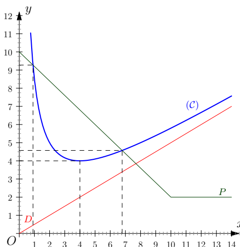
FIGURE 65.2 – Représentation graphique
