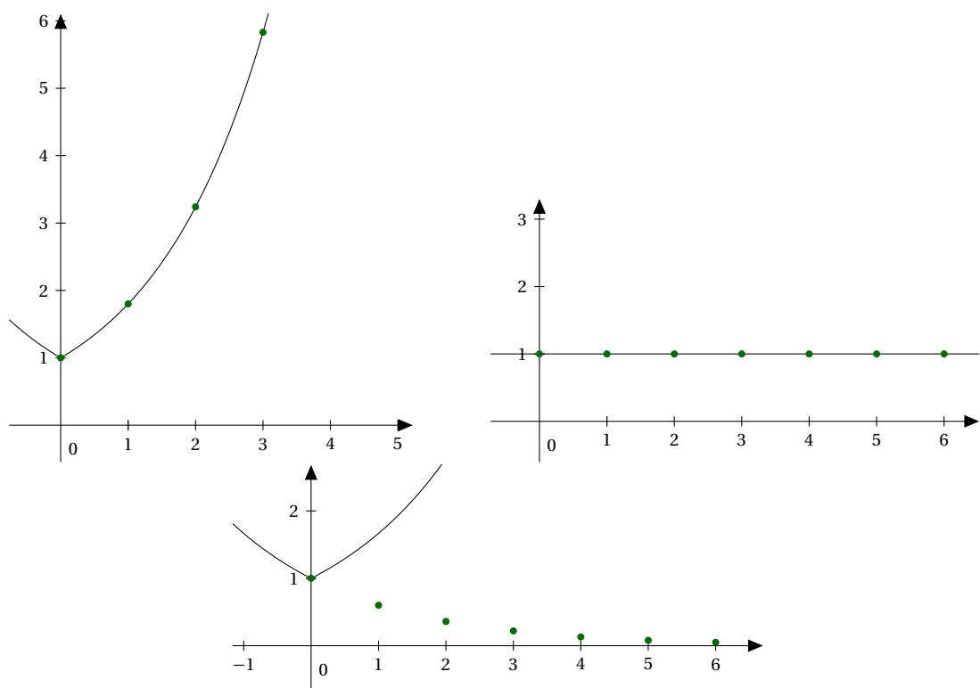
FIGURE 44.1 – Représentation graphique de la suite u_n = a^n avec a > 1 , a = 1 et a < 1
