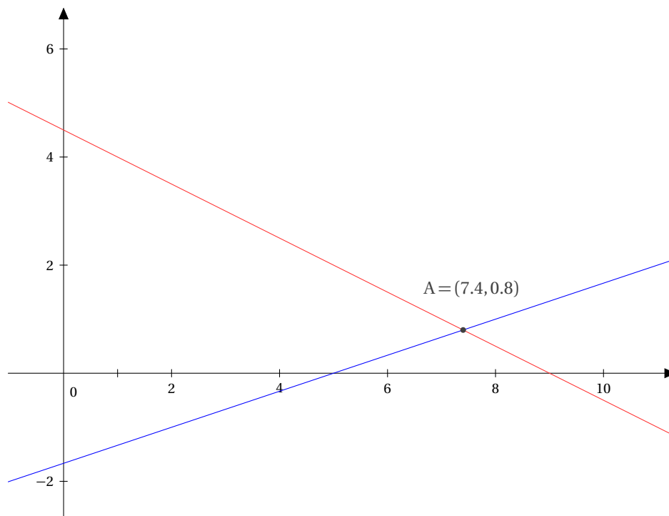
FIGURE 23.1 – Résolution graphique
