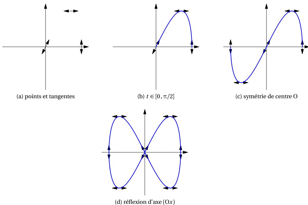
FIGURE 54.3 – Construction de la courbe paramétrée t \mapsto (\cos t, \sin 2t)
