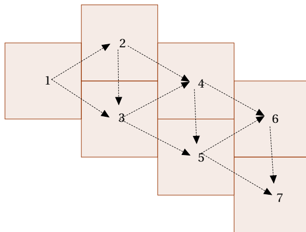
FIGURE 46.4 – Parcours dans un couloir infini
