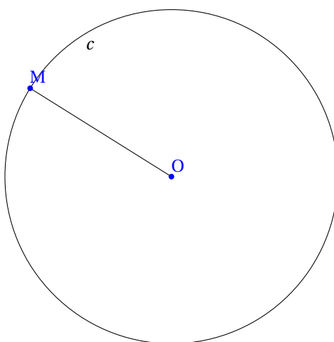
FIGURE 27.1 – Cercle de centre O et de rayon OM
