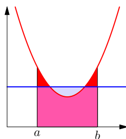
FIGURE 66.16 – Valeur moyenne
