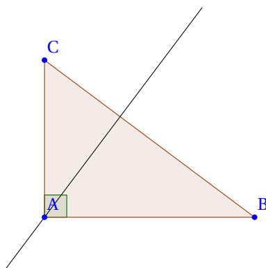
FIGURE 26.5 – Deux des hauteurs d'un triangle rectangle sont confondues avec deux des trois côtés.
