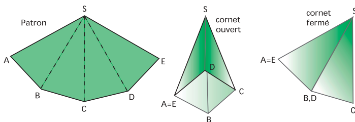
Figure 1. La construction d'une pyramide en carton. Dépouillé de la base ABCDA, cet objet est flexible.
