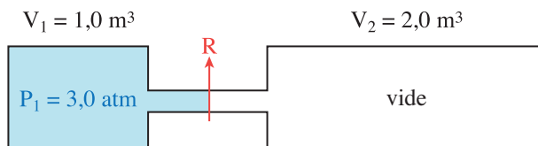
Figure 3.4 – Représentation schématiques des enceintes (1) et (2).
