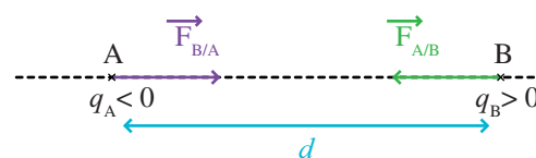
Figure 2.3 – Force exercée par la charge ponctuelle A sur la charge ponctuelle B.
