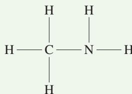
Figure 8.3 – Formule développée de la molécule \text{CNH}_5 .
