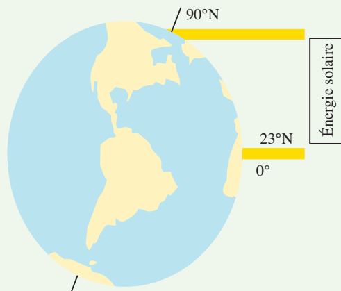
Figure 4.10 – Ensoleillement de l'hémisphère nord au solstice d'été
