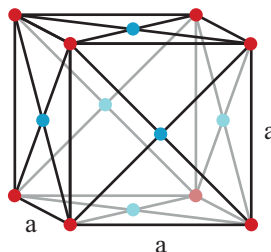
Figure 2.5 – Représentation cubique faces centrées. 8 atomes sont situés aux sommets du cube et 6 atomes au centre de chaque face
