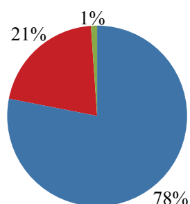
Composition de l'air
