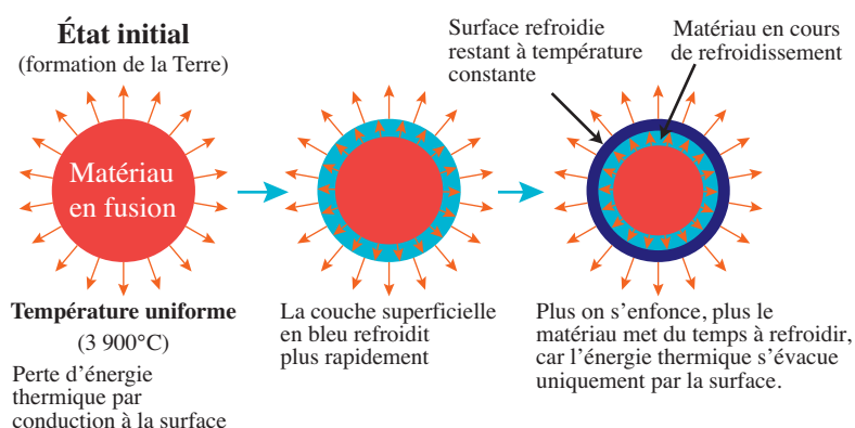
Figure 9.1 – Hypothèse de travail de lord Kelvin
