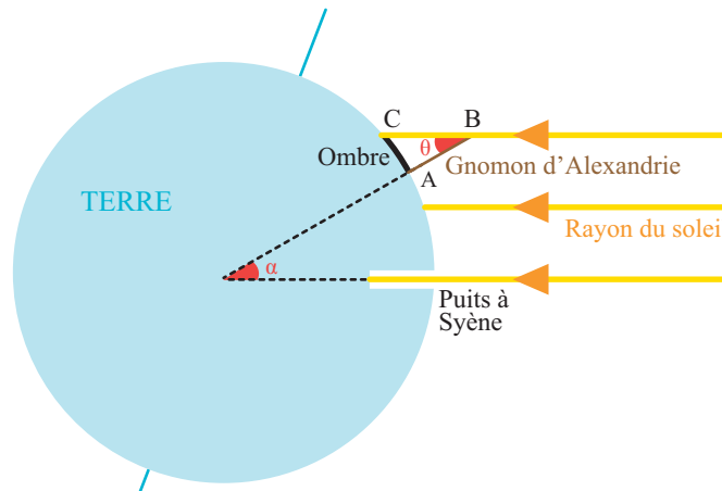
Figure 8.1 – L'expérience d'Ératosthène
