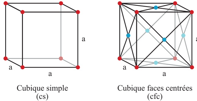
Figure 2.2 – Représentation cubique simple (à gauche) et cubique faces centrées CFC (à droite)
