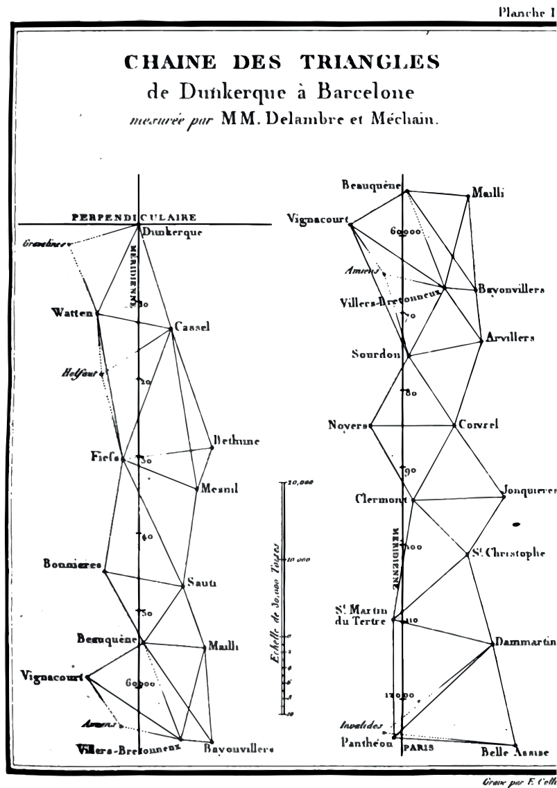
Figure 8.3 – Illustration des triangles de Delambre et Méchain
