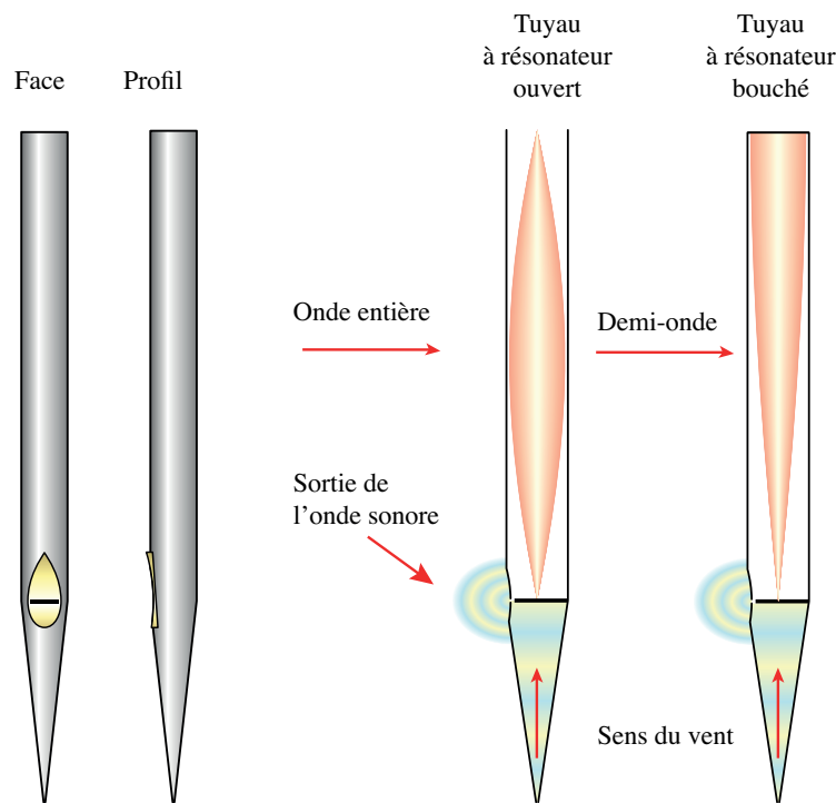
Figure 11.7 – Production du son dans un tuyau d'orgue
