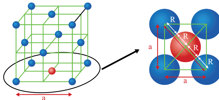
Figure 2.6 – Réseau cubique faces centrées et paramètre de maille
