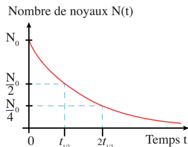
Figure 1.6 – Décroissance radioactive
