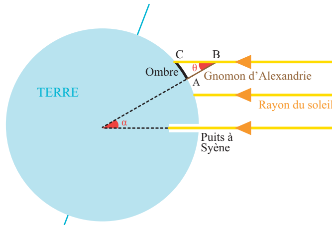
Figure 8.1 – L'expérience d'Ératosthène
