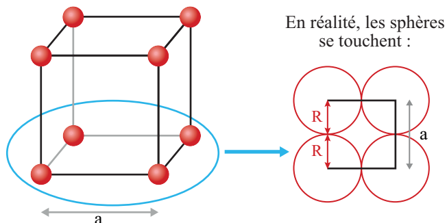
Figure 2.4 – Réseau cubique simple et paramètre de maille
