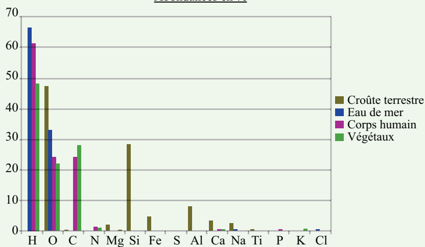
Abondances en %
