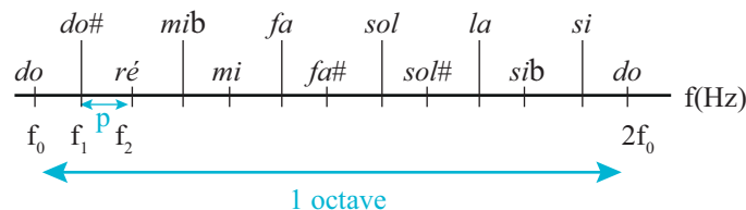
Figure 12.1 – Gamme tempérée
