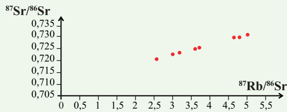
Figure 4.20 – Datation du granite par la méthode Rubidium-Strontium
