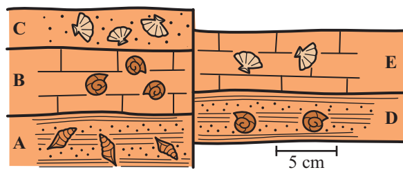
Figure 4.4 – Principe d'identité paléontologique
