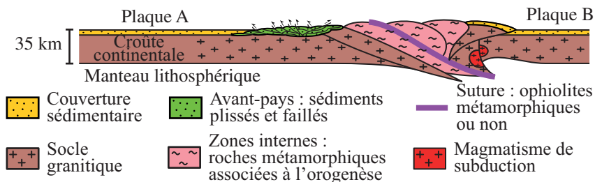
Figure 5.11 – Coupe schématique à travers une ceinture orogénique typique
