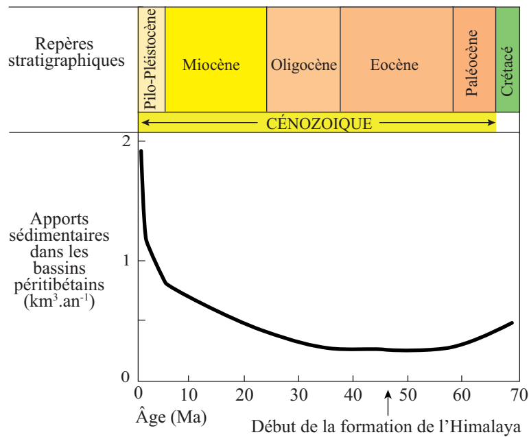
Figure 5.22 – Variations des apports de sédiments par les rivières dans les bassins périthibétains depuis 70 millions d'années
