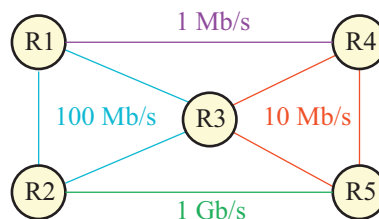
Figure 9.4 – Graphe correspondant au réseau
