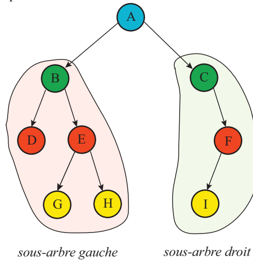
Figure 6.3 – Représentation des sous-arbres gauche et droit de la racine
